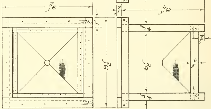
Fly Trap
